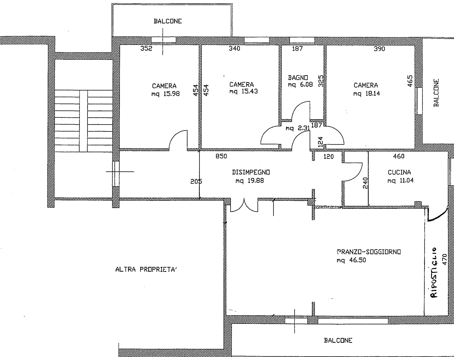
PLANIMETRIA STATO DI FATTO SCALA 1.100 APPARTAMENTO MQ. 157.53
